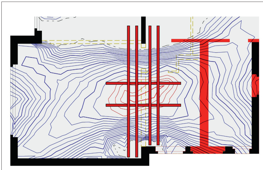
Durch «re-plate» lassen sich der Biege- und Schubwiderstand erhöhen sowie die Durchbiegungen reduzieren. Die re-fer AG bietet bei Bedarf Bemessungshilfen an. (Im Bild: schematische Darstellung der Verstärkung)
