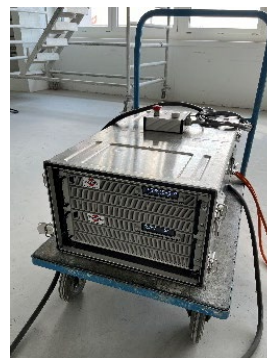
Heizgerät elektrische Widerstandsheizung (nur durch re-fer Techniker CH)
